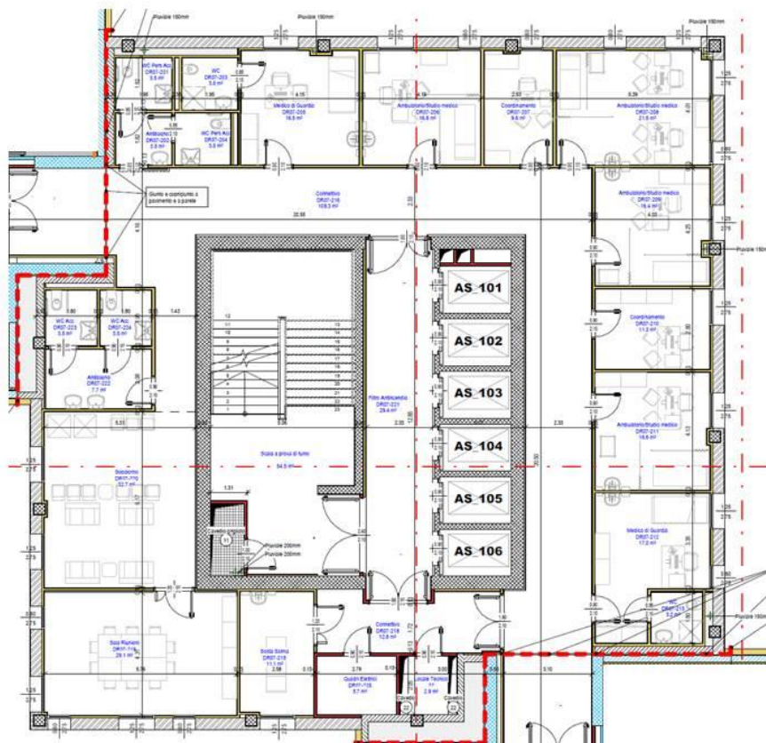
Planimetria del piano tipo (liv.7)
